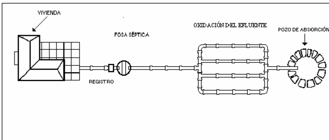
FIGURA 1. SISTEMA DE TRATAMIENTO FOSA SEPTICA (figura ilustrativa)
